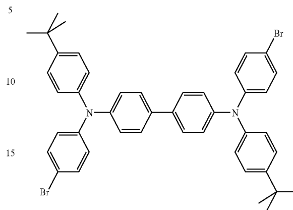
Monomer M5
