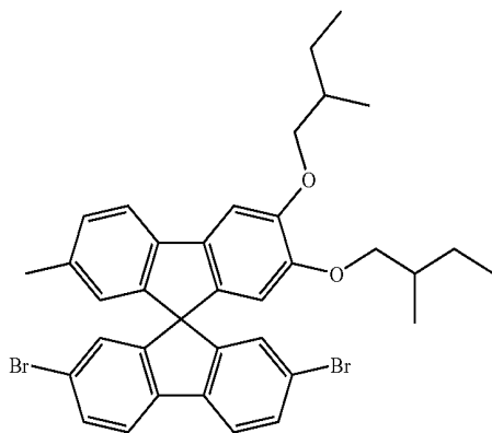
Monomer M3
