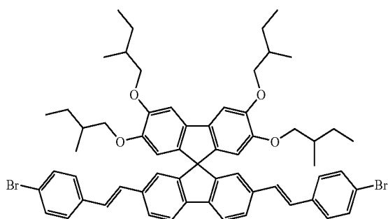
Monomer M4
